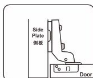
HBE33C Insert 内藏
