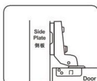
HBE34C Insert 内藏
