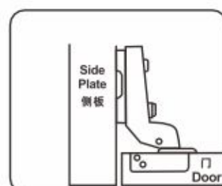
HB109C Insert 内藏
