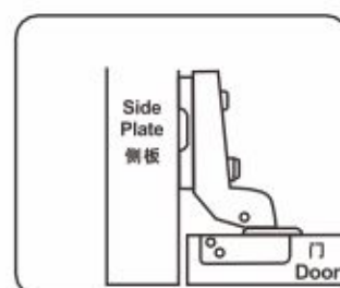
HB1784C Insert 内藏
