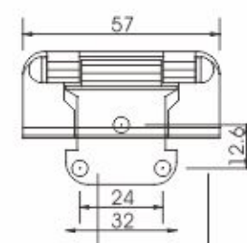
HS101 Up door spring hinges 上翻门支撑铰链
