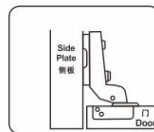
HBS183C Insert 内藏
