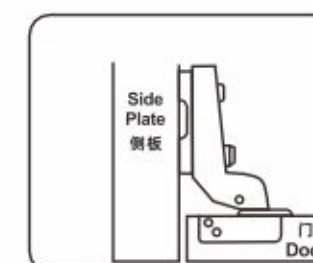
HB127C Insert 内藏
