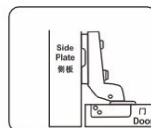
HB183C Insert 内藏
